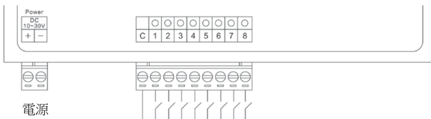
圖 2-7 警報信號配線圖
