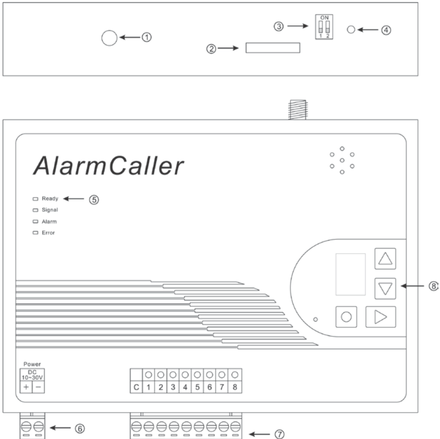
圖 2-1 AD340-DI1V/DI8V 簡訊報警機的零件名稱
