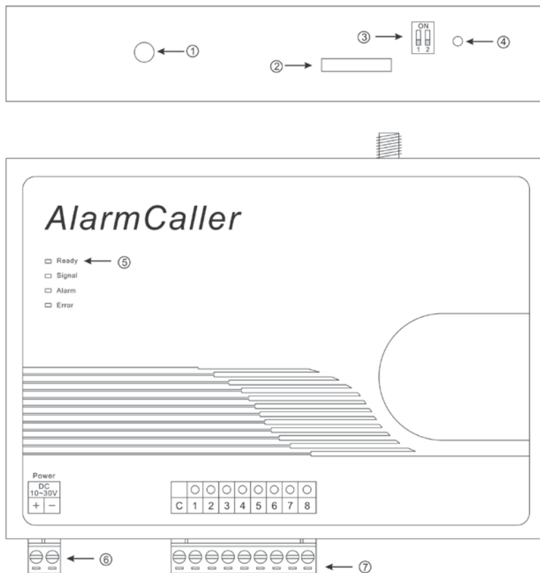
圖 2-1 AD340-DI1/DI8 簡訊報警機的外觀與零組件名稱
