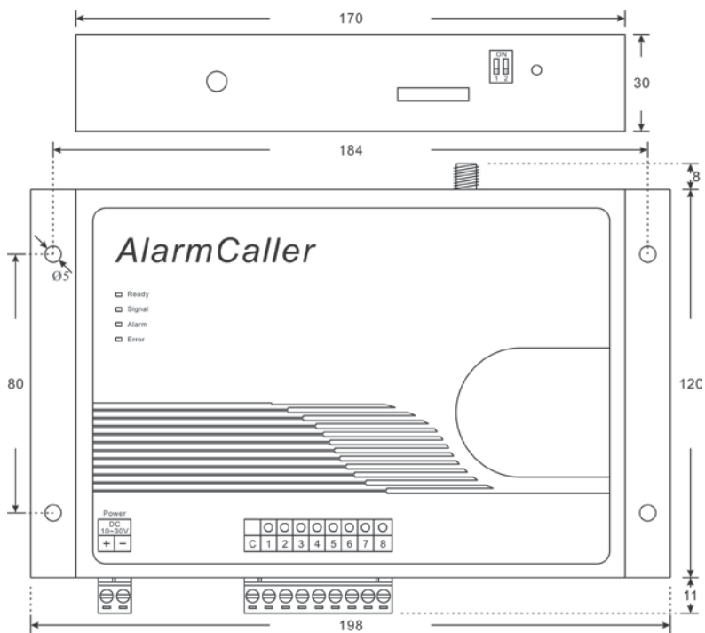
圖 2-2 AD340-DI1/DI8 簡訊報警機的外觀尺寸
