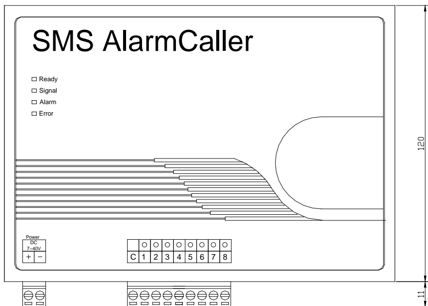
圖 2-2 簡訊報警機 AD310-SCF 外觀尺寸
