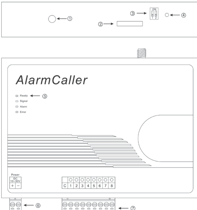
圖 2-1 簡訊報警機 AD310-SCF 外觀及零組件名稱
