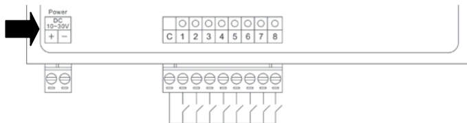
圖 2-6 電源接線
