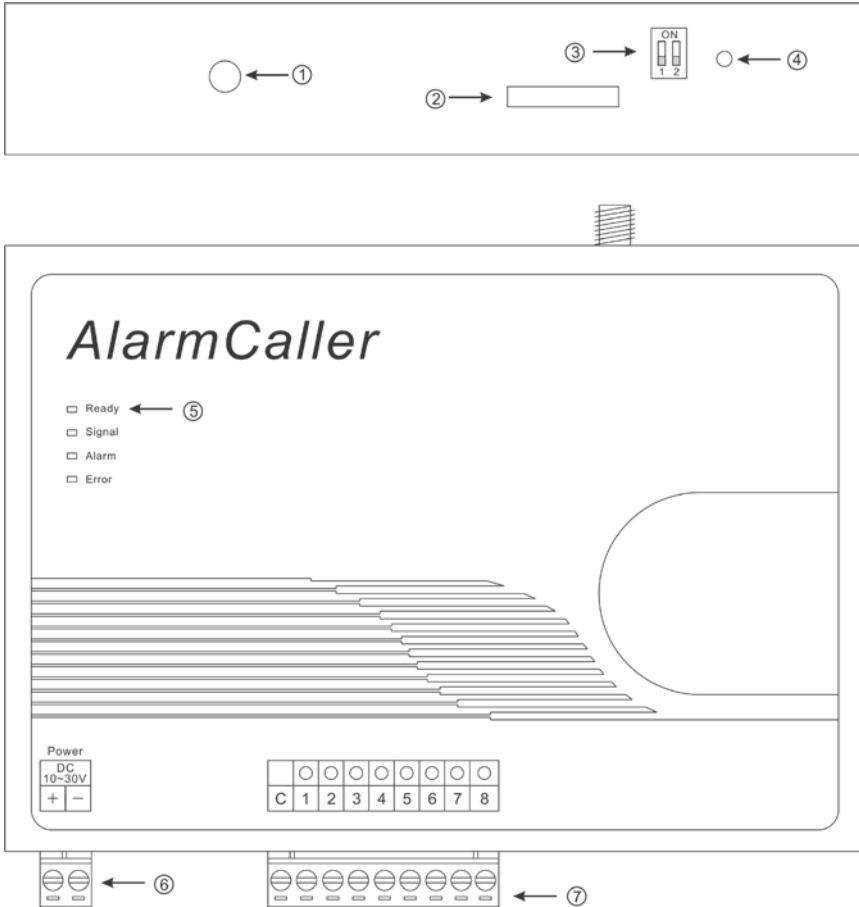
圖 2-1 簡訊報警機 AD310-CI64MS 外觀及零組件名稱
