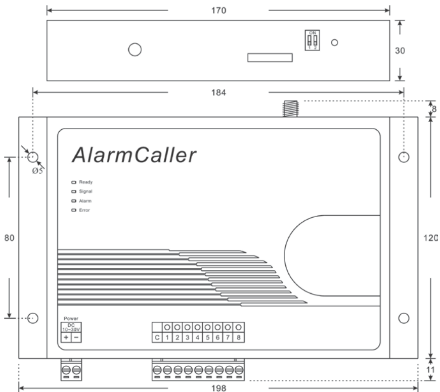
圖 2-2 簡訊報警機 AD310-CI64MS 外觀尺寸
